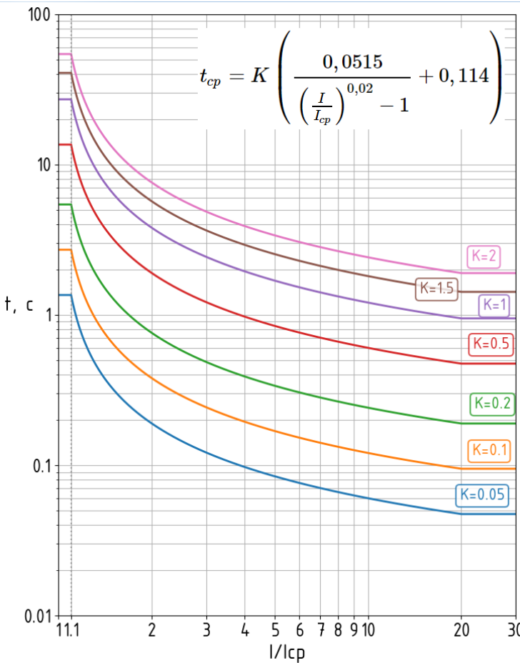
Рисунок И.4 – Кривая D (Умеренно инверсная ANSI)
